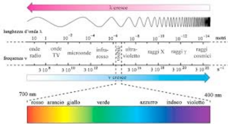
Figura 1: Rappresentazione dello spettro elettromagnetico, che mette in evidenza la porzione relativa alla "luce visibile" percepita dall'occhio umano.
